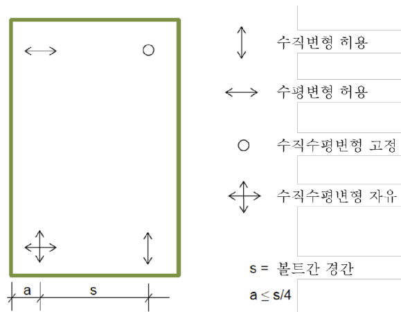
[그림 4.4-1] 유리판 볼트접합의 허용 면내변형 방향
